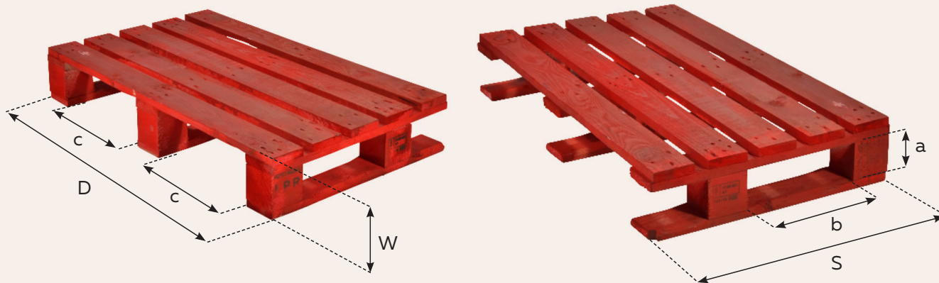
DP610 - Nominalne wymiary i tolerancja palety (mm)
